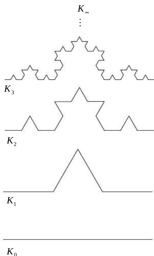
図2 コッホ曲線
