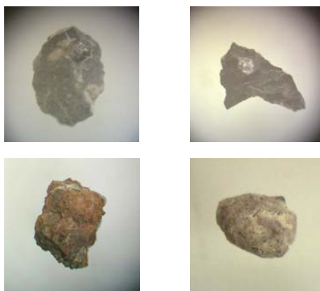
図2 火山灰中に含まれていた鉱物
