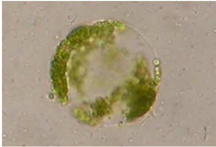
図1 ホウレンソウのプロトプラスト
