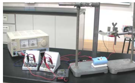
図1 実験装置
