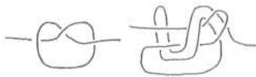
図1 2つの「結び目」
