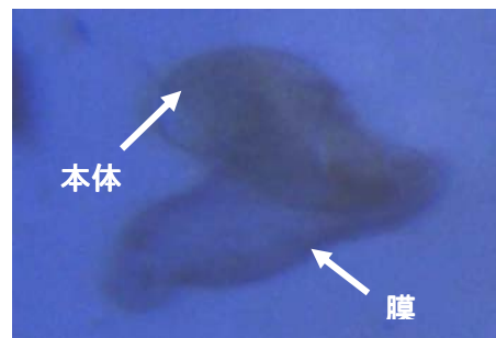
図6 メチルグリーンピロニン
