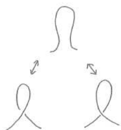
①ライデマイスター移動Ⅰ
