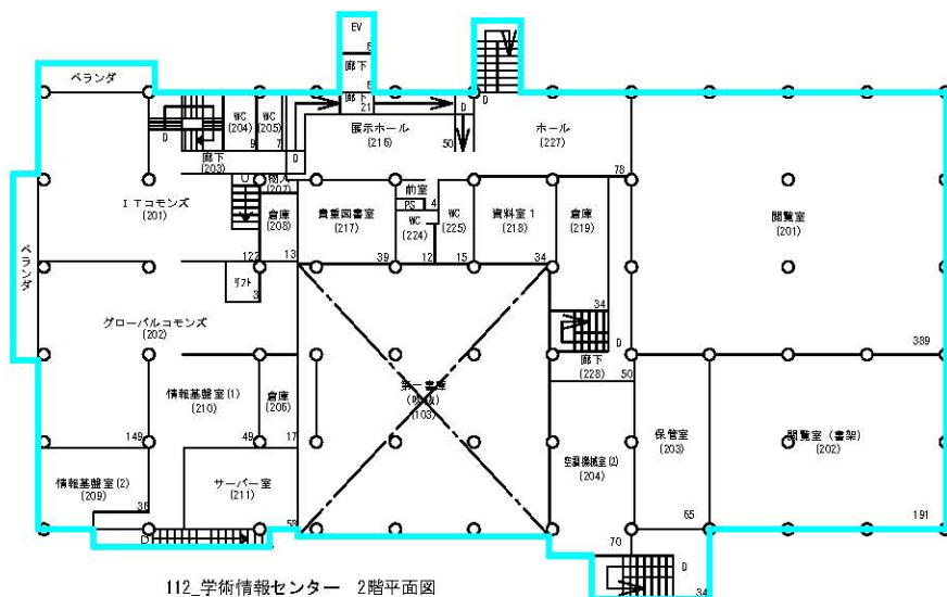
112_学術情報センター 2階平面図
