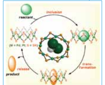
有機小分子(シクロヘキサノン)を包摂した テトラ型8核パラジウム錯体 と開発中の触媒反応
