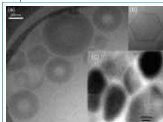
両親媒性化合物がつくる分子集合体。 (a)ドーナツ型凝集体、(b)多角形ベシクル、 (c)多重層ベシクル
