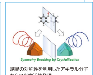
結晶の対称性を利用したアキラル分子からの光学活性発現
