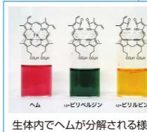
生体内でヘムが分解される様子
