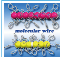
直鎖上ナノクラスター(分子性金属錯)
