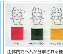
生体内でヘムが分解される様子
