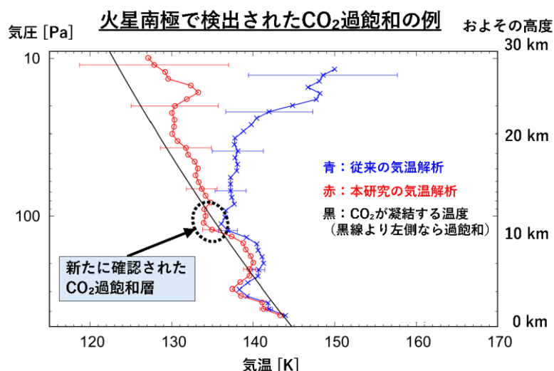
図：火星南極の極夜で観測された気温データの例。この例では、従来の気温解析（青）では検出できなかったCO 2 過飽和層が、高度約11 km付近で新たに確認されたことを示している。
