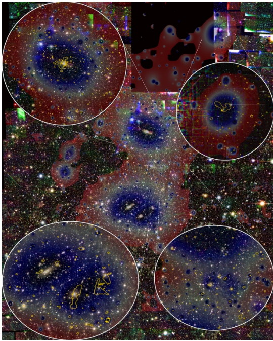
図 4 DECам カメラで撮影したアーベル 3391/95 銀河団の可視光画像。eROSITA 画像（黒や青などはガス密度が高い場所）と ASKAP 望遠鏡の電波の等高線（黄色）が重ねて表示されている。© Reiprich et al. Astronomy & Astrophysics
