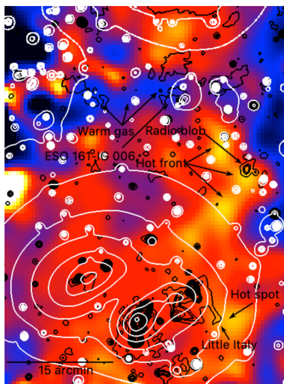
図 3 アーベル 3391/95 の南北の銀河団をつなぐ「橋」の拡大図。電離した酸素の輝線放射が見えやすいエネルギー帯に絞って表示してある。白色の等高線は eROSITA 望遠鏡の X 線画像、黒色の等高線は ASKAP/EMU 望遠鏡の電波画像。青色が、温かいガス(Warm gas)からの酸素輝線放射が強い領域。黄色はガス温度が高い場所で、「リトル イタリア(Little Italy)」や「電波ブロッブ (Radio blob)」などのラベルがついた電波放射が強い場所とも近い。© Reiprich et al. Astronomy & Astrophysics
