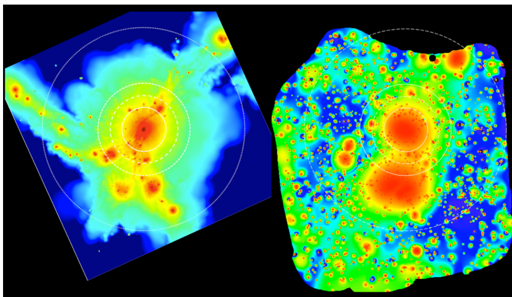
図2 eROSITA による X 線画像 (右) と比較のためのシミュレーション画像(左) 右図では、過去の観測では検出できなかったガスの非常に希薄な領域も見てとれる。北側の銀河群から銀河団 A3391、A3391 と A3395 の間、さらに A3395 から南の小さな銀河群へとつながる長さ 5000 万光年のガスフィラメントが存在することがわかる。©左: Reiprich et al. Space Science Reviews , 17, 195; 右: Reiprich et al. Astronomy & Astrophysics
